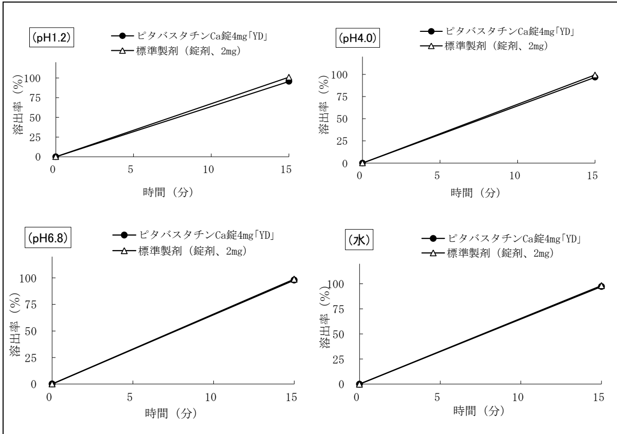
判定時点での試験製剤の溶出率
