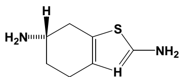
類縁物質 A(原薬由来)
