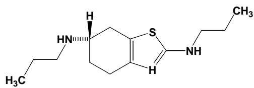
類縁物質 B(原薬由来)
