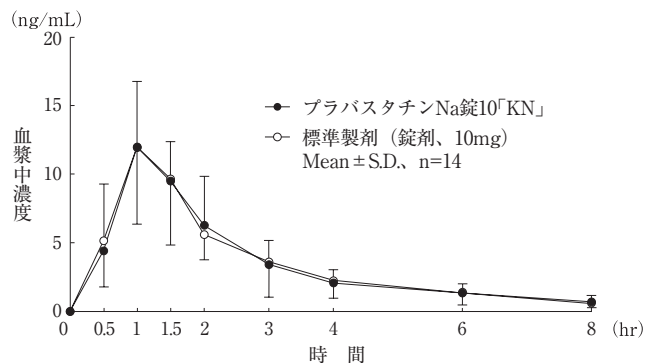
図2 10mg投与時のプラバスタチンナトリウム血漿中濃度推移
