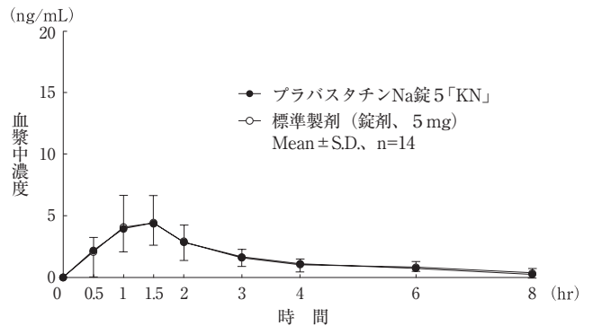
図1 5mg投与時のプラバスタチンナトリウム血漿中濃度推移
